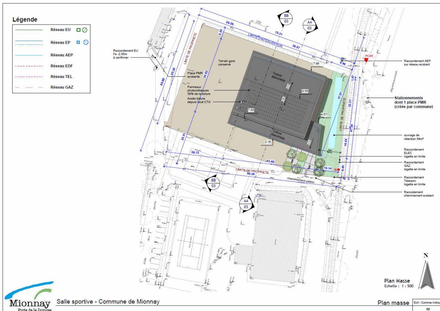
Figure 3 – Plan de masse de la future salle sportive de MIONNAY
