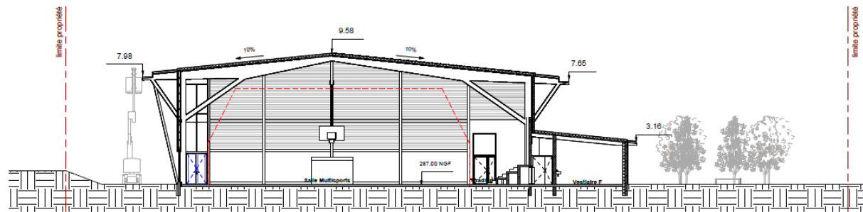
Coupe AA'
