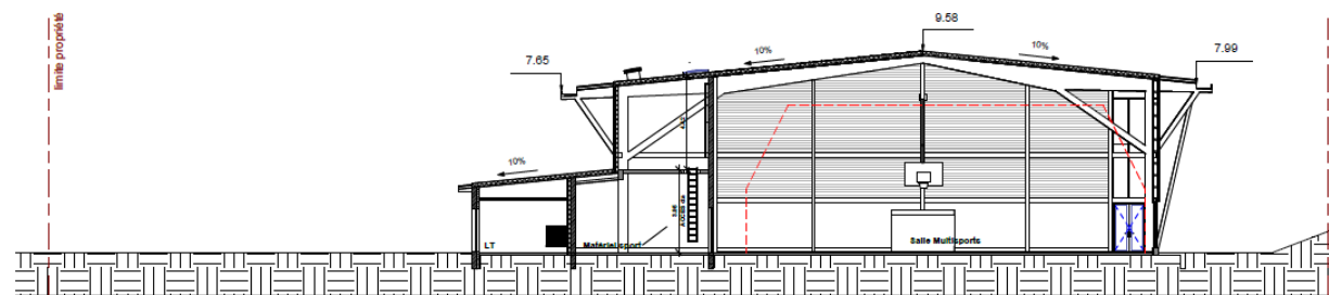
Coupe BB'
